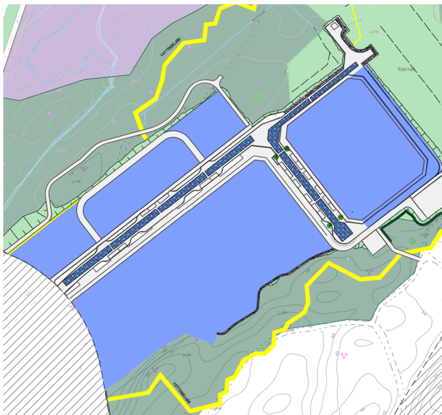
Bild 20: Översikt principlösning med makadambäddar (blå stråk) för kvartersdagvattnets rening i gatorna.
