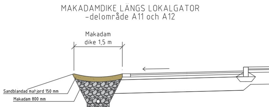
Bild 9: Ytledes avledning till makadamdike föreslås vid mindre trafikerade lokalgator. Sandblandad matjord i ytskiktet och underliggande makadam.
