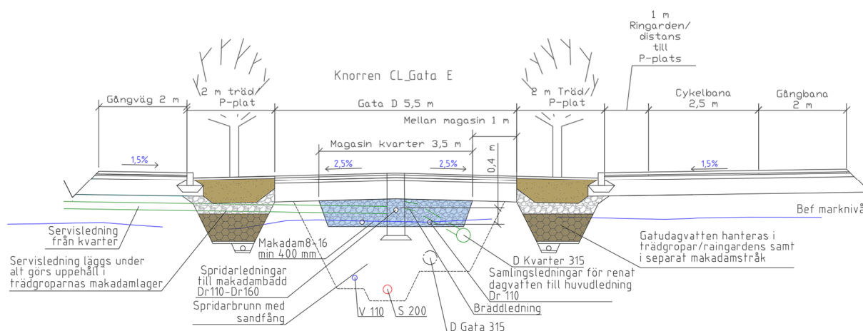
Bild 21: Principsektion för gata E. Underjordiska makadambäddar för kvartersdagvatten under överbyggnaden i gatan. Trädgropar med makadambäddar för gaturdagvatten längs gatans båda sidor. De renande anläggningarna hålls separerade och avleds/bräddas till varsin huvudledning.
